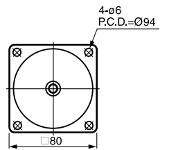
⑨ 4GN-10X 重量 0.45kg
