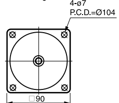
⑫ 5GN-10X 重量 0.6kg
