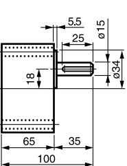
⑭ 5GU-3~180 KB 重量 1.3kg (60, 90, 120W 共用)
