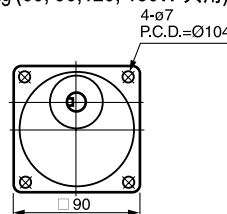
⑭ 5GU-3~180 KB 重量 1.3kg (60, 90, 120, 150W 共用)
