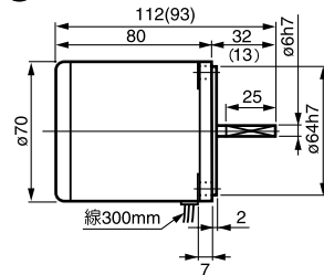
④ 3IK15A(GN)-□ 重量 1.1kg
