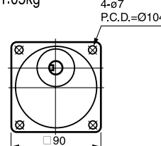
⑪ 5GN-3~18 L=42 重量 0.7kg (40~150W 共用) 5GN-20~180 L=58 重量 1.05kg
