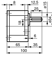
⑰ 5GU-3~180 K 重量 1.3kg (60, 90, 120W 共用)
