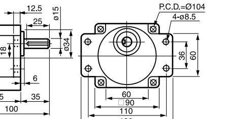
⑰ 5GU-3~180K 重量 1.3kg (60, 90, 120W 共用)
