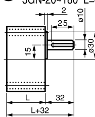
⑤ 3GN-3~18 L=32 重量 0.45kg 3GN-20~180 L=42 重量 0.55kg
