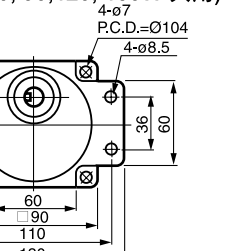
⑰ 5GU-3~180K 重量 1.3kg (60, 90, 120, 150W 共用)
