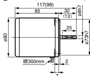
⑦ 4IK25A(GN)-□ 重量 1.6kg
