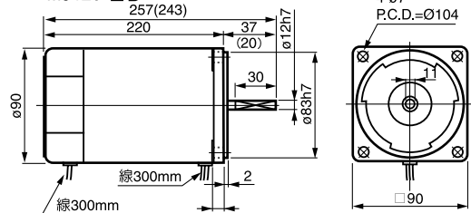
⑯ M590-□B 重量 4kg M5120-□B
