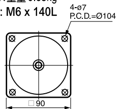
⑮ 5GU-10XK 重量 0.65kg 適用螺絲: M6 x 140L
