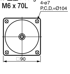
⑱ 5GU-10XKS 重量 0.65kg 適用螺絲: M6 x 70L
