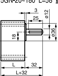
⑪ 5GN-3~18 L=42 重量 0.7kg (40~120W 共用) 5GN-20~180 L=58 重量 1.05kg
