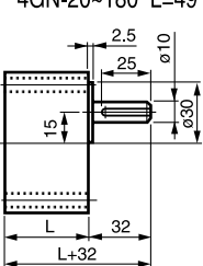
⑧ 4GN-3~18 L=35.5 重量 0.5kg 4GN-20~180 L=49 重量 0.7kg
