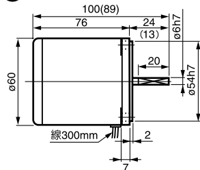
① 2IK6A(GN)-□ 重量 0.7kg
