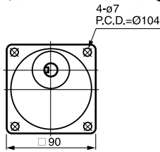
⑭ 5GU-3~180 KB 重量 1.3kg (60, 90, 120W 共用)
