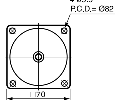
⑥ 3GN-10X 重量 0.35kg
