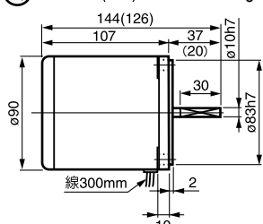
⑩ 5IK40A(GN)-□ 重量 2.5kg
