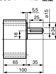
⑭ 5GU-3~180 KB 重量 1.3kg (60, 90, 120, 150W 共用)
