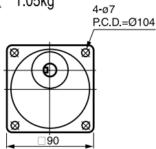
⑪ 5GN-3~18 L=42 重量 0.7kg (40~120W 共用) 5GN-20~180 L=58 重量 1.05kg
