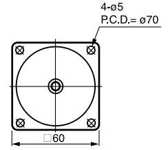
③ 2GN-10X 重量 0.3kg
