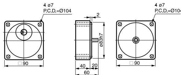
⑨ 5GU-10XK 重量 0.65kg 適用螺絲: M6 x 140L
