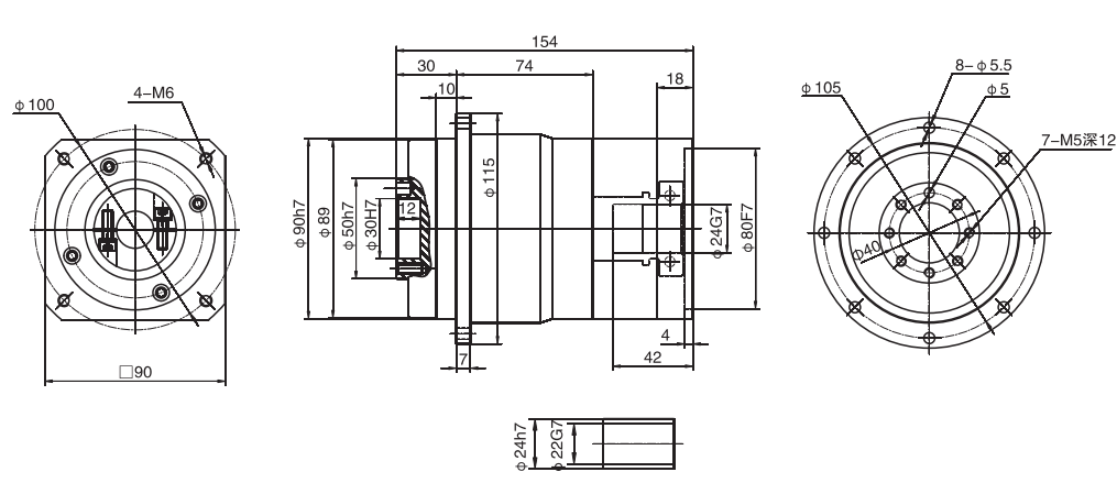
WPLH90雙級 / Double stage
