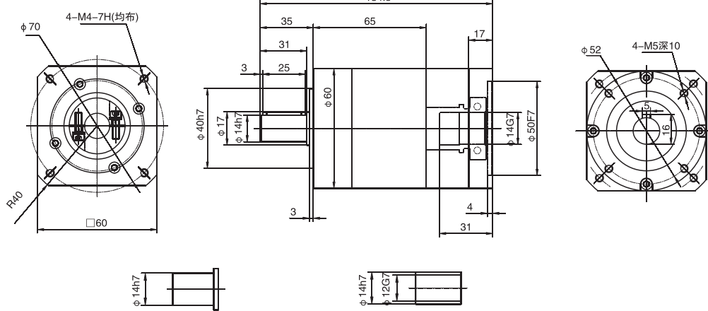
WPL60雙級 / Double stage
