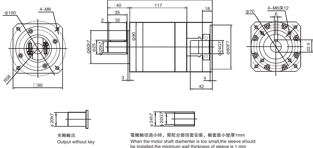
WPL90三級 / Three stage
