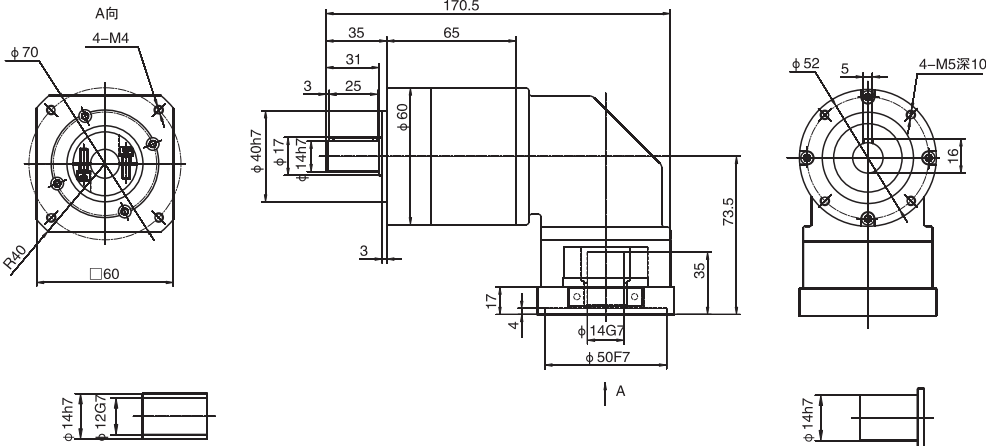
WPLR60雙級 / Double stage
