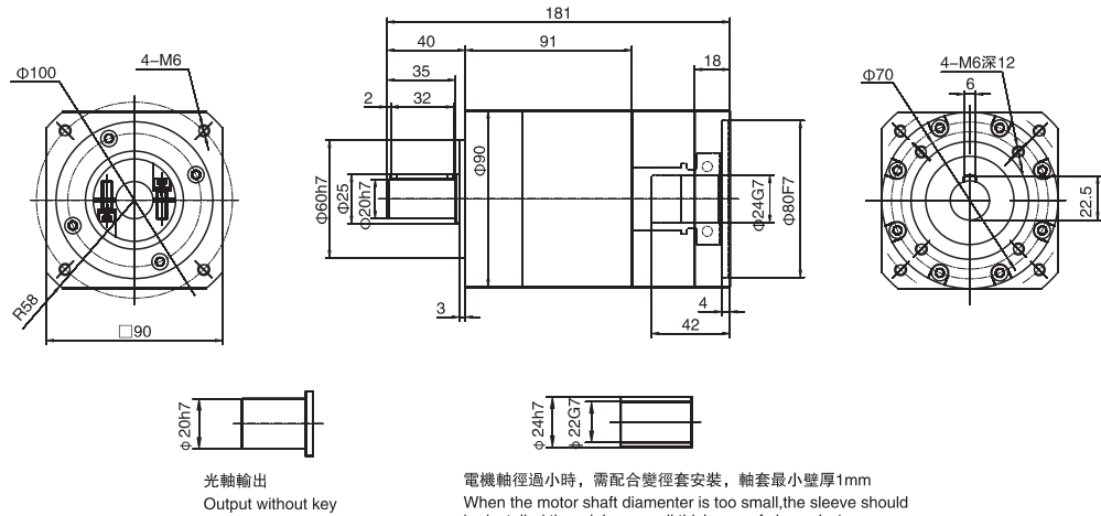
WPL90雙級 / Double stage
