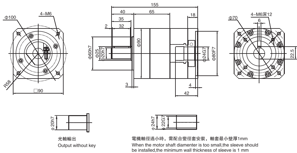
WPL90雙級 / Double stage
