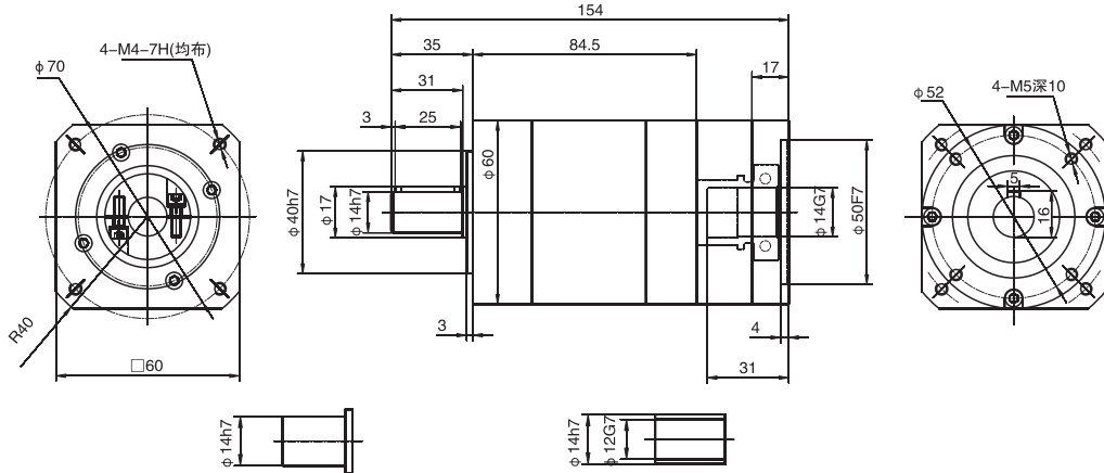
WPL60三級 /Three stage
