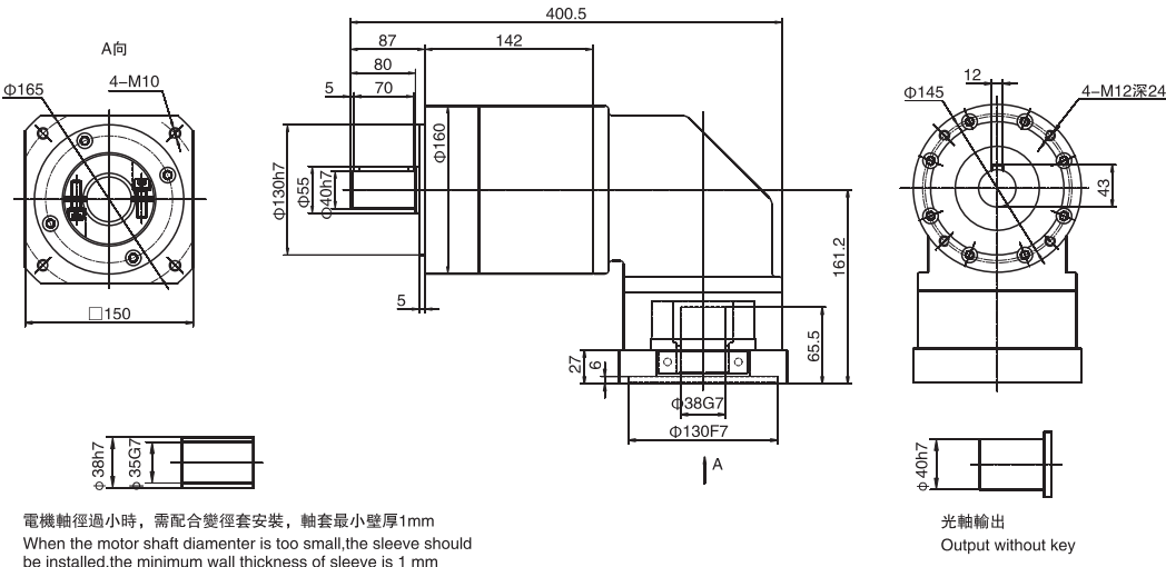
WPLR160雙級 / Double stage
