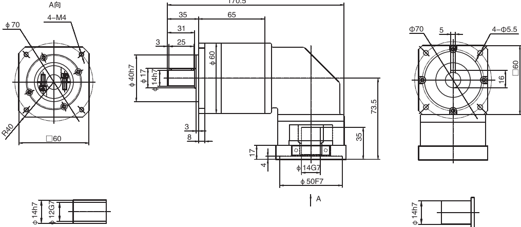
WPLFR60雙級 / Double stage
