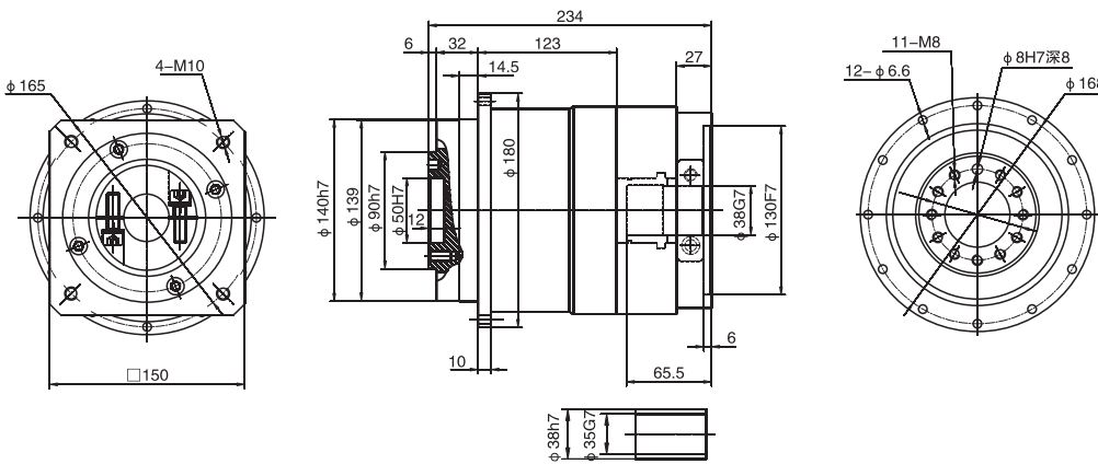
WPLH160雙級 / Double stage
