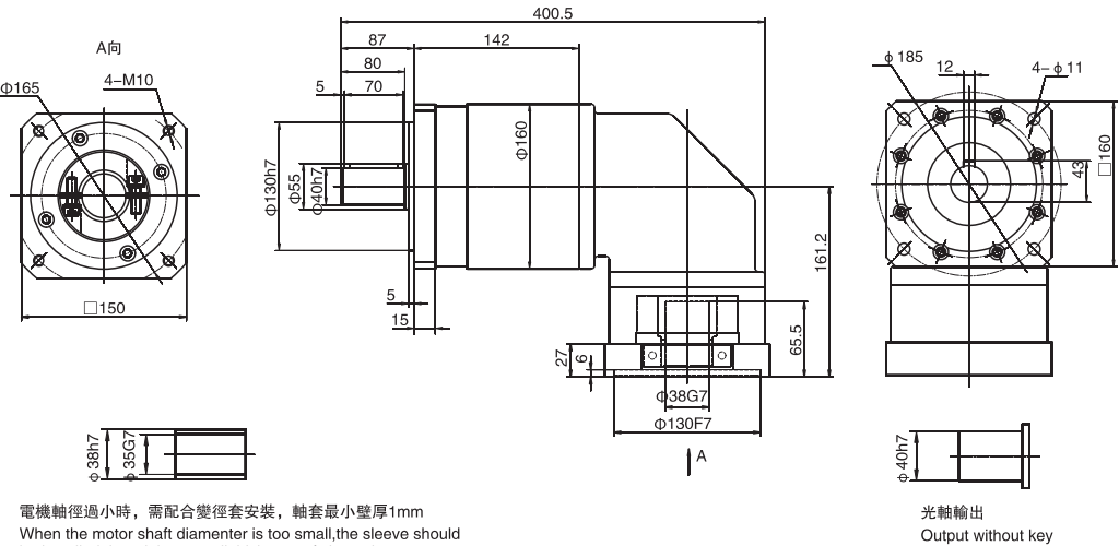
WPLFR160雙級 / Double stage
