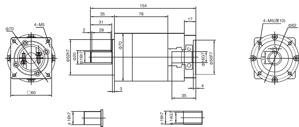
WPL70雙級 / Double stage
