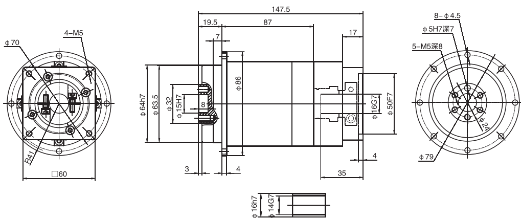
WPLH70三級 / Three stage
