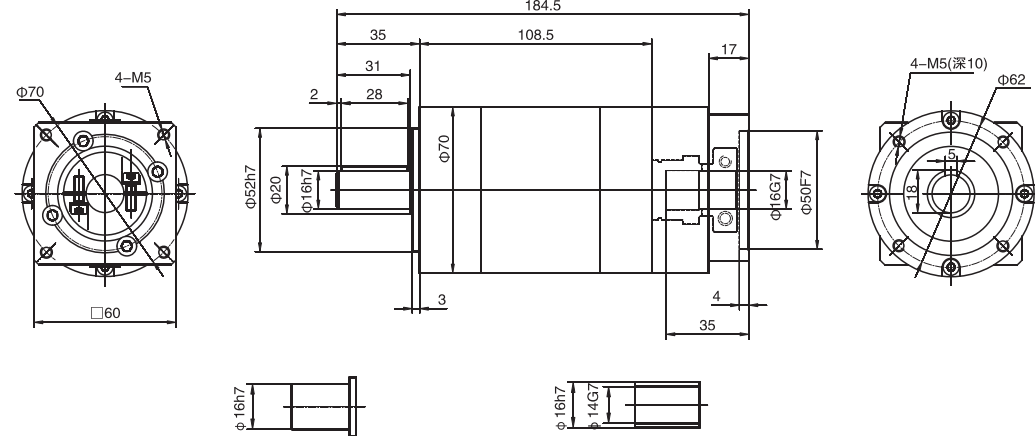
WPL70三級 /Three stage
