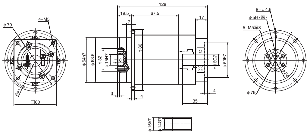
WPLH70雙級 / Double stage
