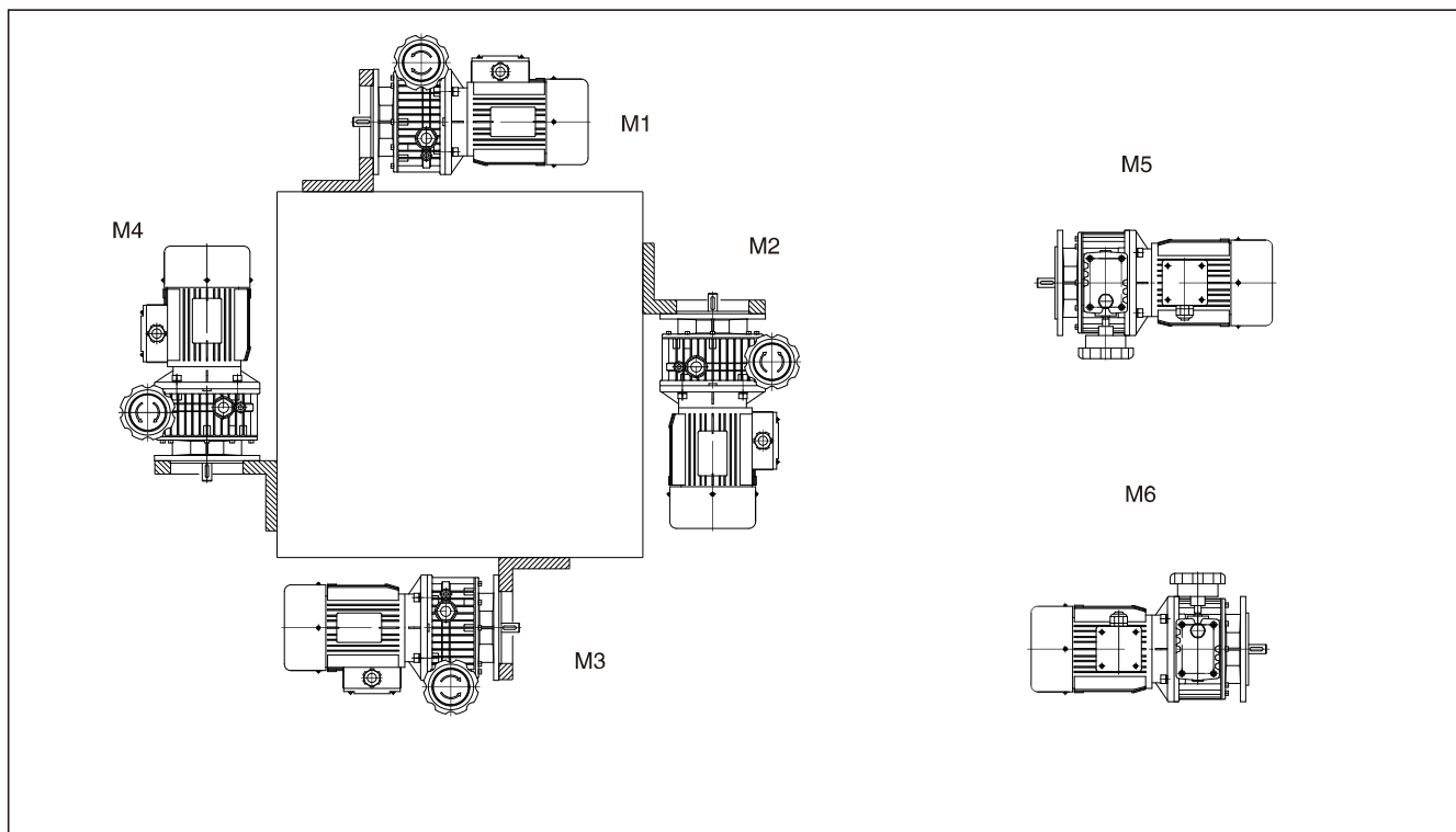
MBF无级变速机安装方式
