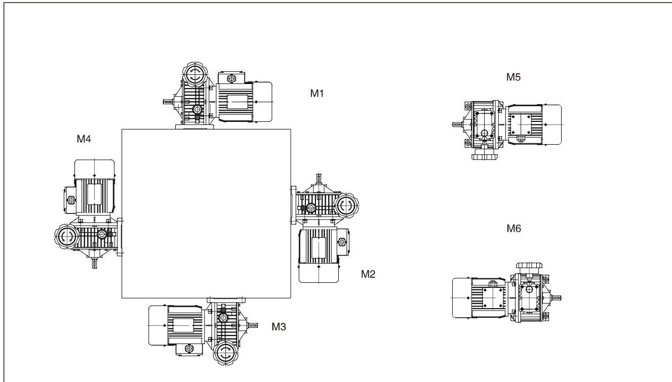
MBW无级变速机安装方式
