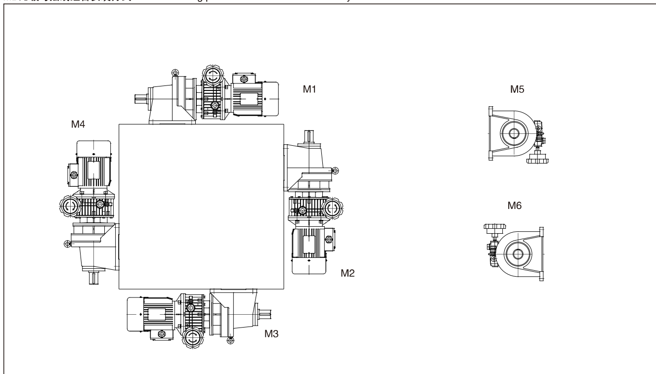
MB无级与摆线组合安装方式
