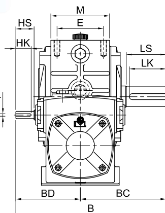
Input Shaft 入力軸
