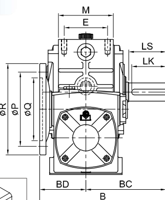
Output Shaft 出力軸
