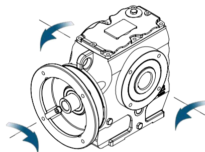
旋轉方向 Rotation Directions
