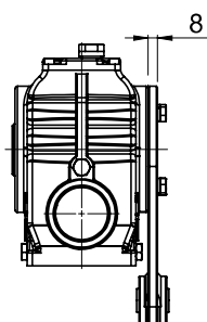
側固型 Torque arm
