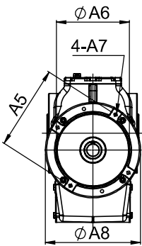
Input Shaft 入力軸
