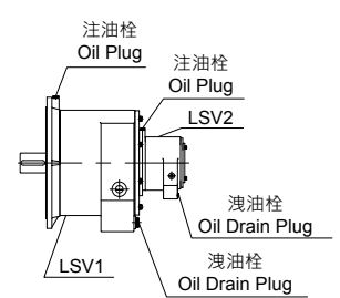
V-OH 立式 - 軸水平 Vertical Type - Shaft Horizontal
